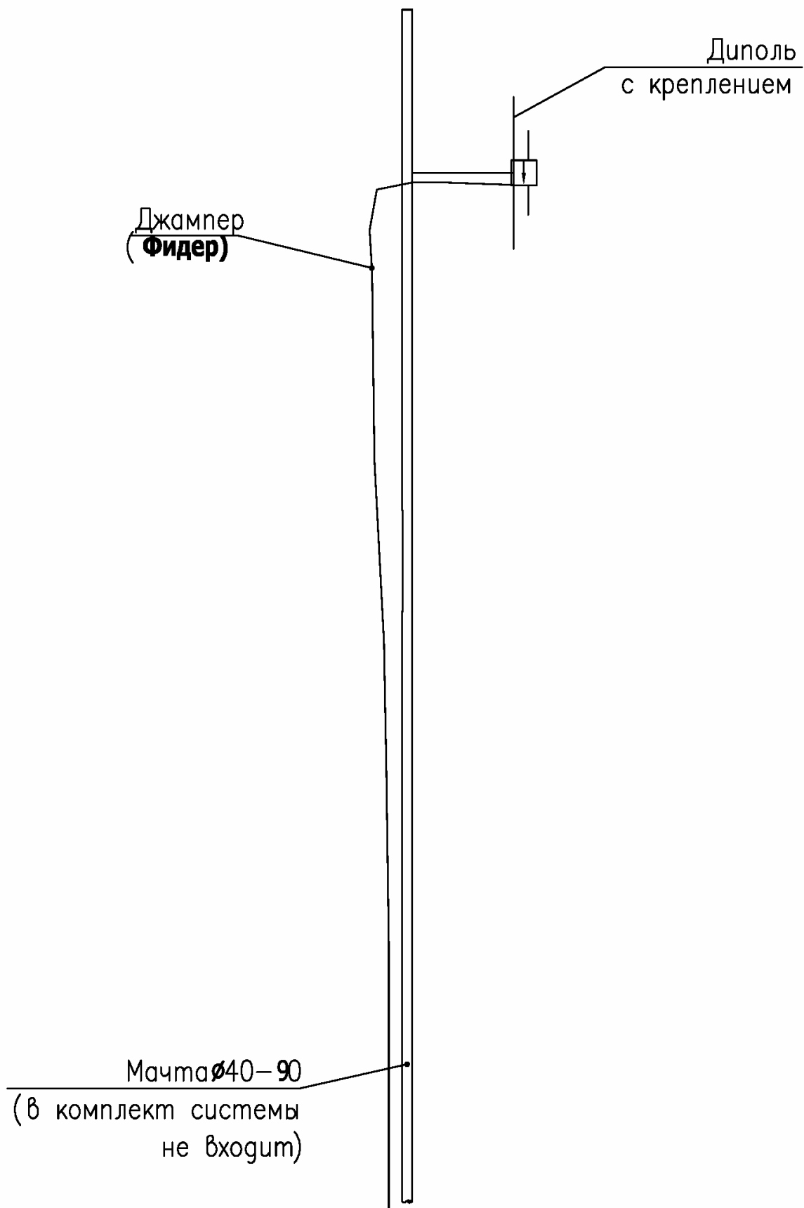
Рис.1 Антенна AFM-D2W
